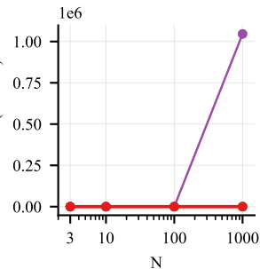
(h) Enzyme/4-state
