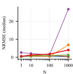
(d) Glycolysis/4-state
