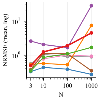
(a) Glycolysis/4-state
