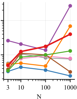
(a) Glycolysis/4-state
