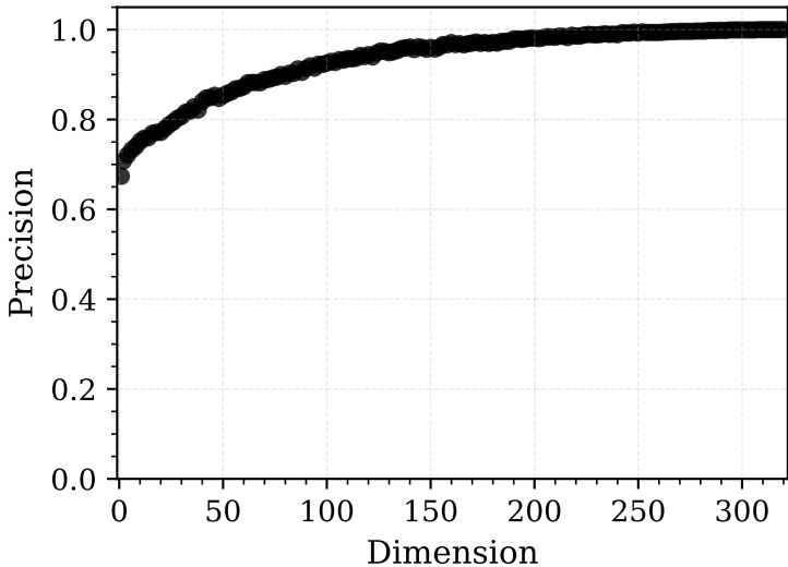
Precision@5
