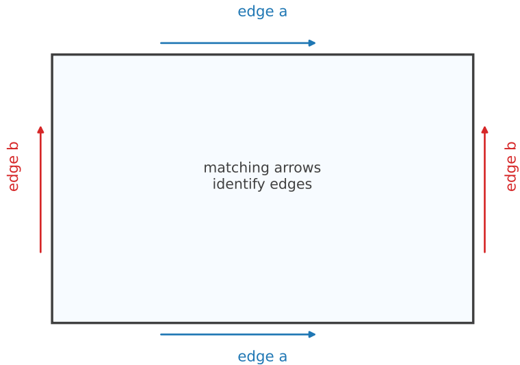
(a) Brillouin torus
