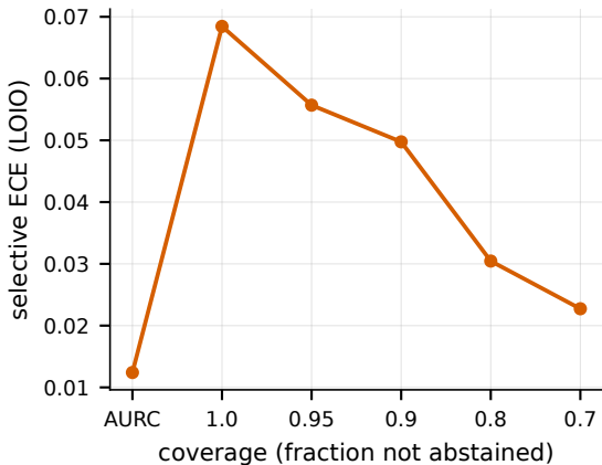
MVTec (full 15)
