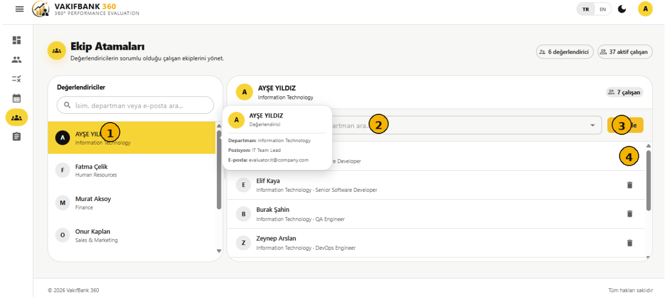
Şekil 5 — Ekip Atamaları. 1: değerlendirici listesi • 2: çalışan arama/seçim • 3: Ekle • 4: atama kaldırma.
