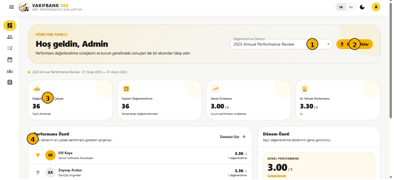
Şekil 2 — Admin ana ekranı. 1: değerlendirme dönemi • 2: Excel aktarımı • 3: özet kartları • 4: performans özeti.
