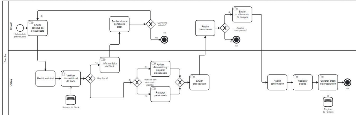
Figura 1: Diagrama BPMN AS-IS — Proceso manual de presupuestación en FerroLux. Diagrama editable disponible en: /docs/to-be.bpmn (abrir con bpmn.io)
