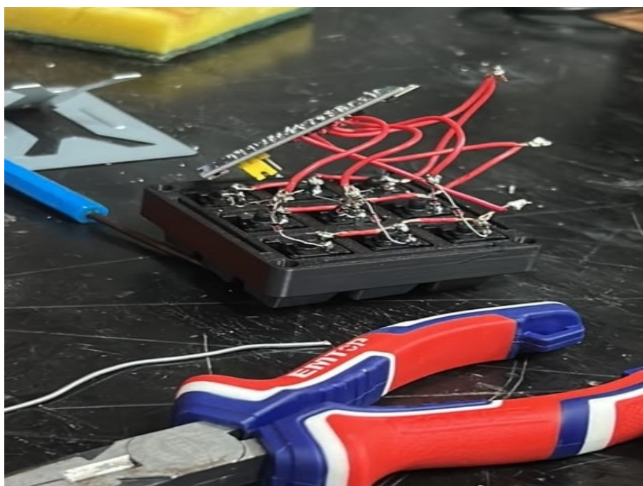
Figura 2 — Processo de soldagem e montagem física dos switches mecânicos e diodos 1N4148.
