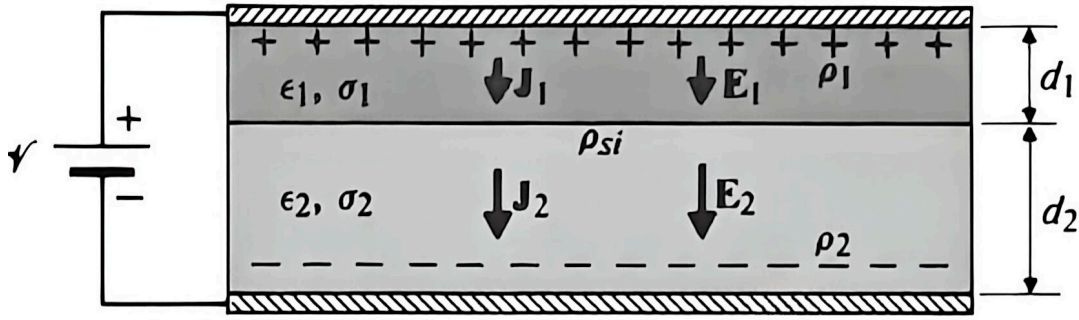
图 5-6-2 层状介质中的恒稳电流分布
