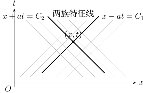
图 3.3: 第一象限中的两族特征线示意图。加粗直线表示经过点 (x, t) 的两条特征线。
