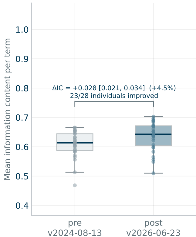
SOCS1 (n = 28)
