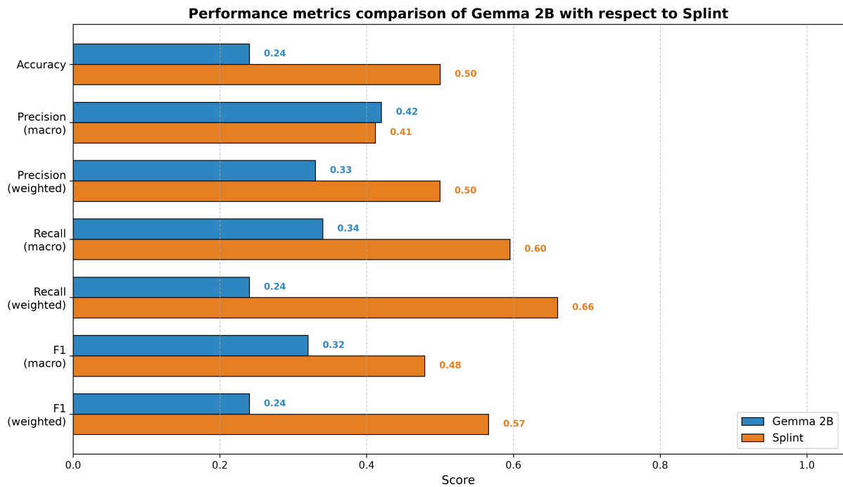
Figura 3: Gráfico de barras con las métricas de rendimiento de Google Gemma 2B en comparación a Splint
