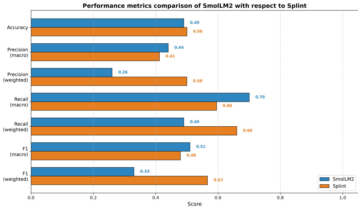
Figura 7: Gráfico de barras con las métricas de rendimiento del ajuste fino de parámetros de Hugging Face SmolLM2 en comparación a Splint
