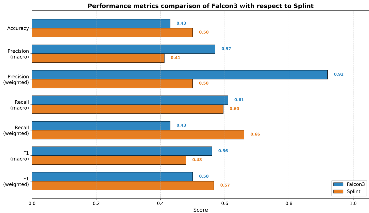
Figura 5: Gráfico de barras con las métricas de rendimiento del ajuste fino de parámetros de Falcon3 en comparación a Splint
