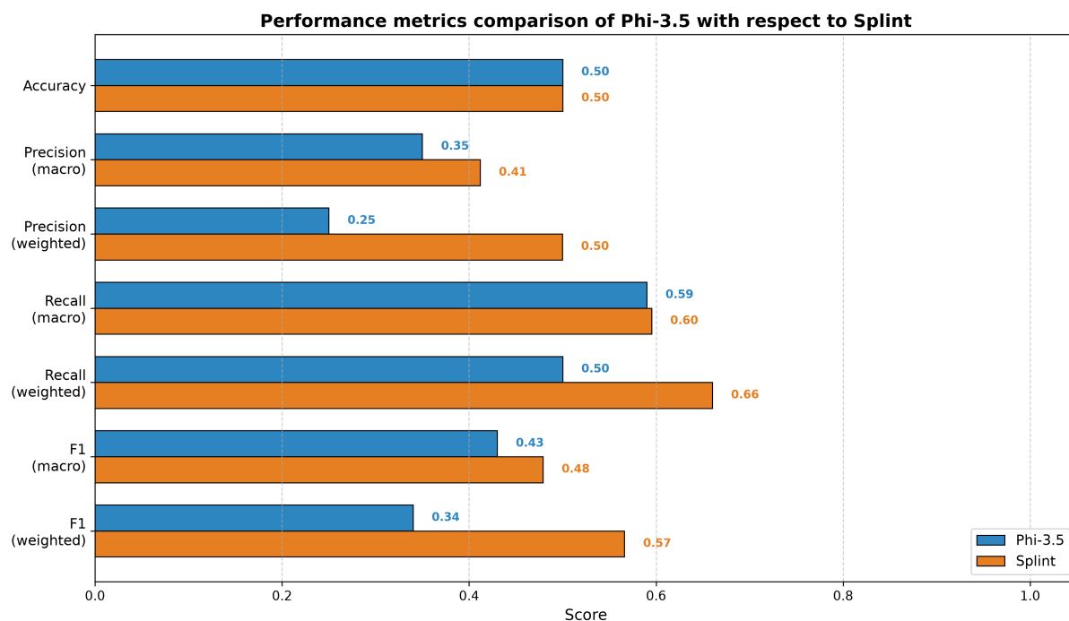
Figura 4: Gráfico de barras con las métricas de rendimiento de Microsoft Phi 3.5 en comparación a Splint
