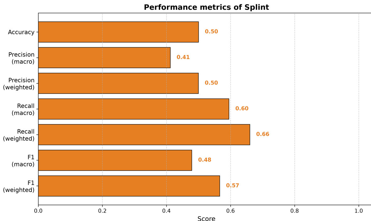
Figura 2: Gráfico de barras con las métricas de rendimiento de Splint
