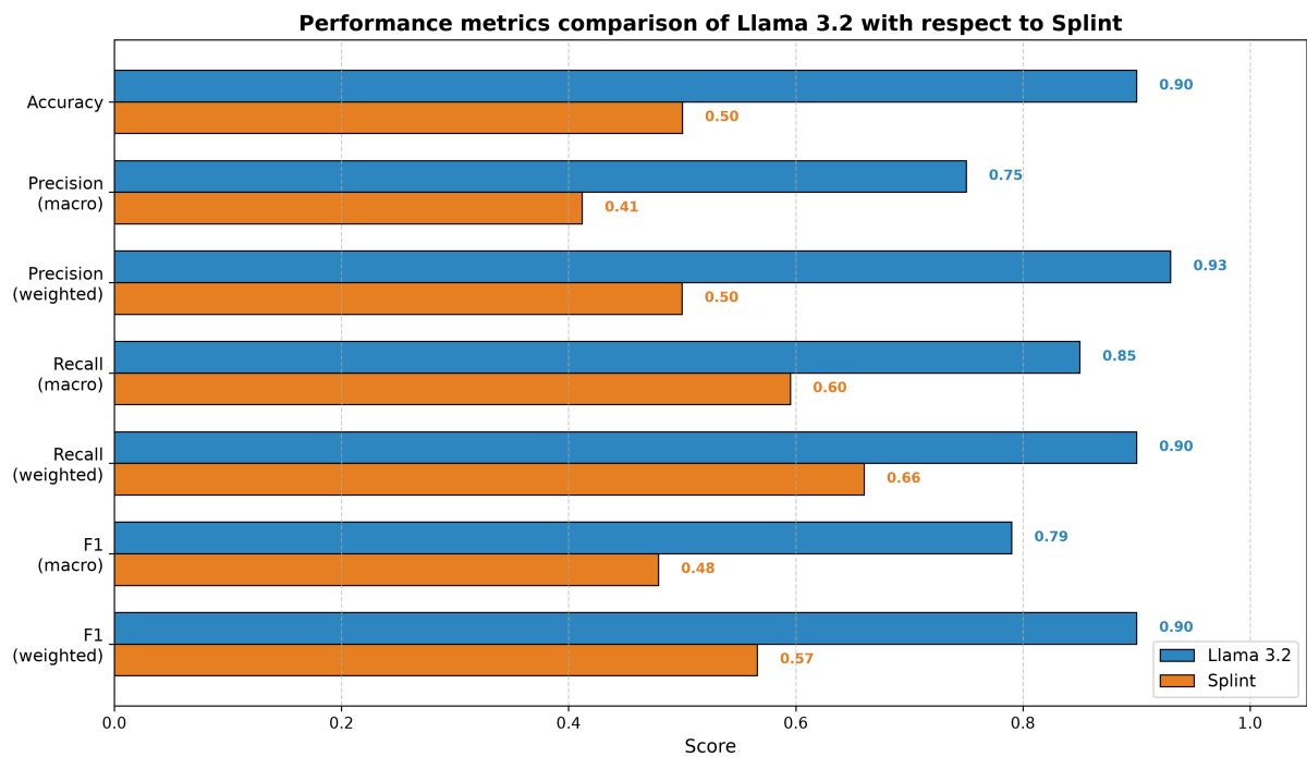
Figura 6: Gráfico de barras con las métricas de rendimiento del ajuste fino de parámetros de Meta Llama 3.2 en comparación a Splint
