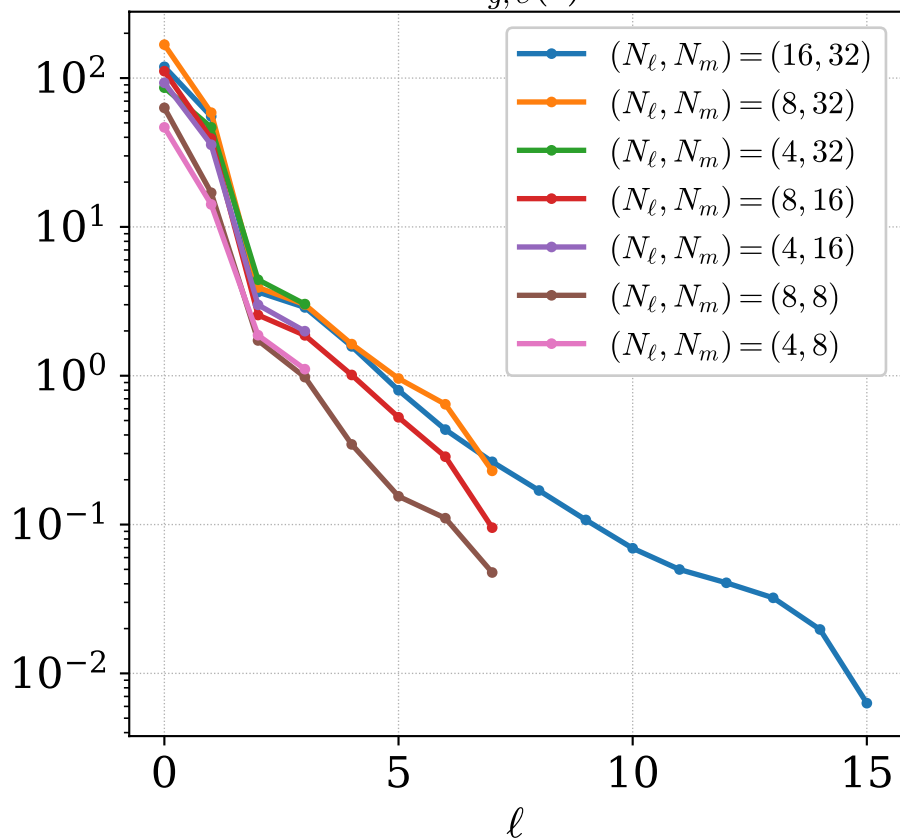
W_{g,e}(\ell)
