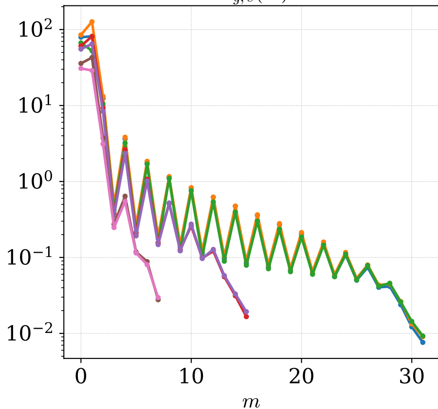
W_{g,e}(m)
