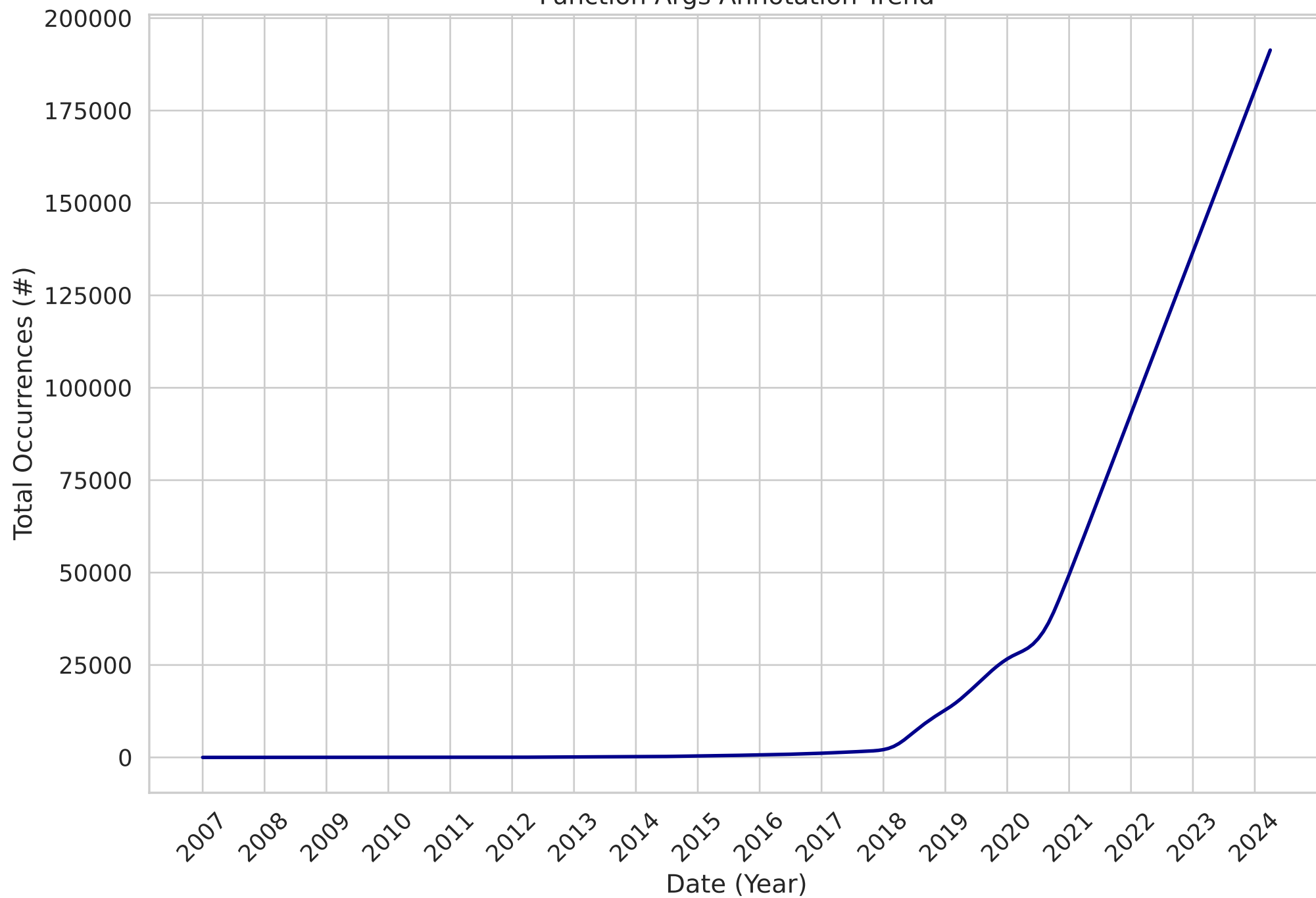
Function Args Annotation Trend
