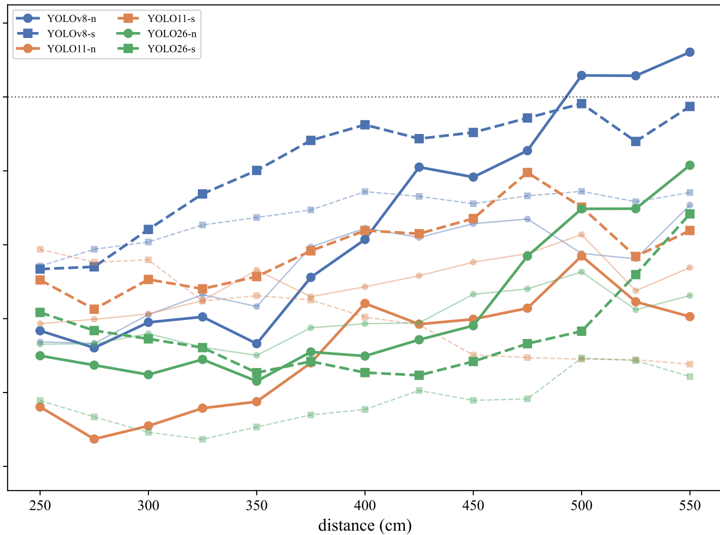
INT8(ModelOpt mixed→excl.cv4)
