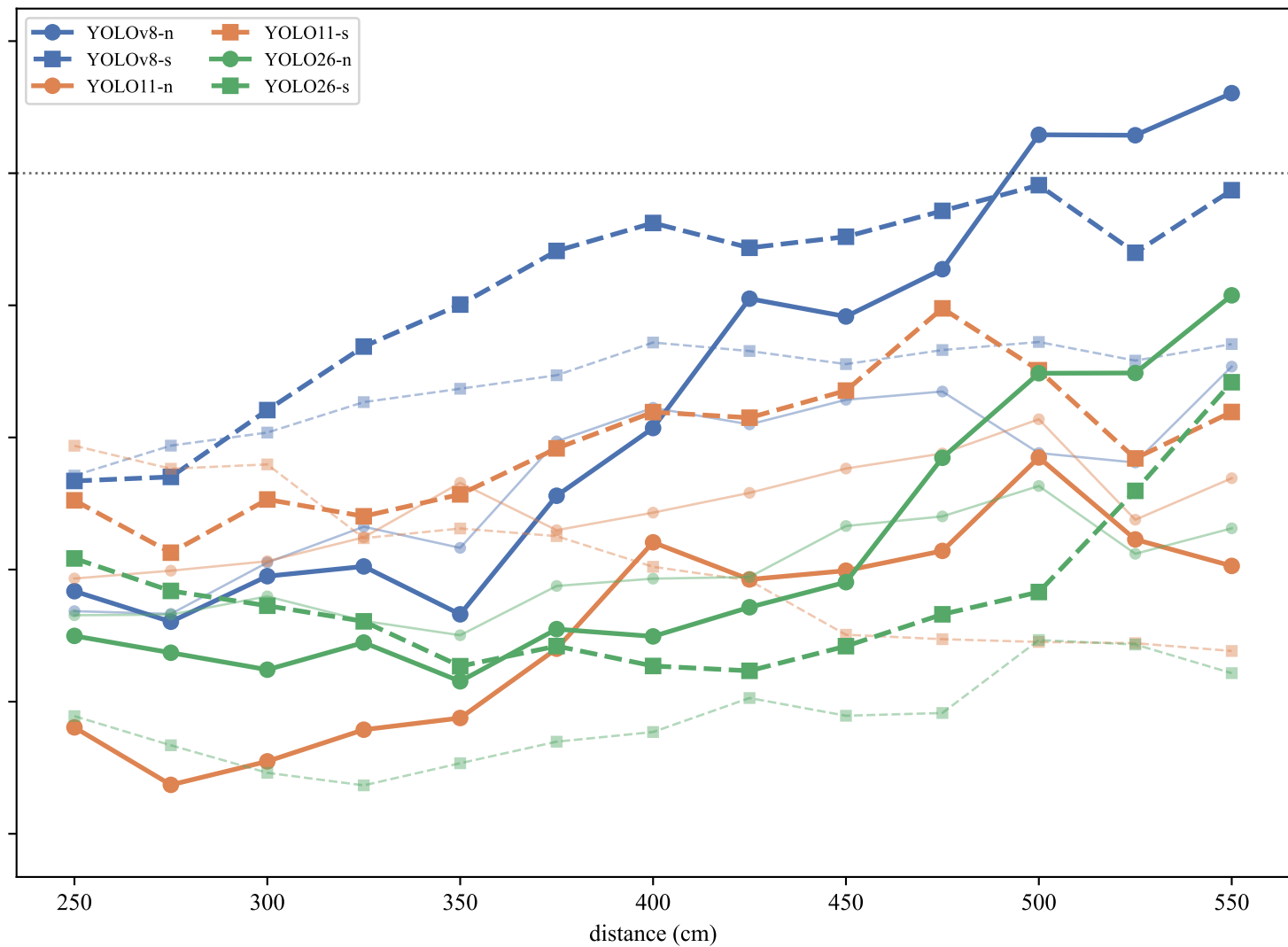
INT8(ModelOpt mixed→excl.cv4)
