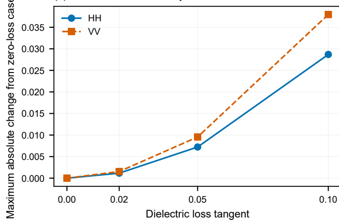
(d) Dielectric-loss sensitivity
