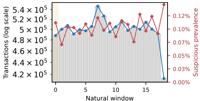
SAML-D
