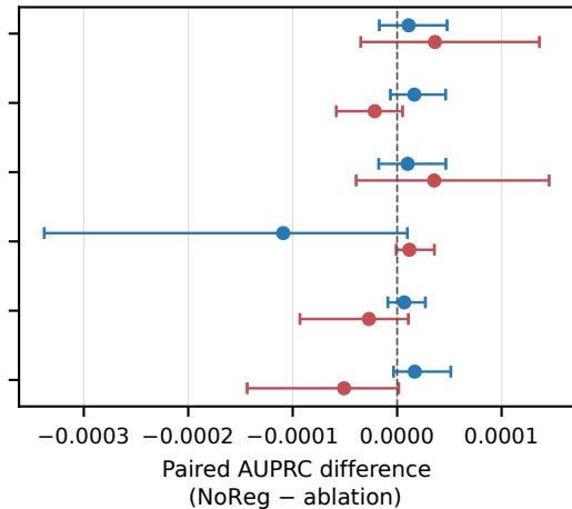
SAML-D
