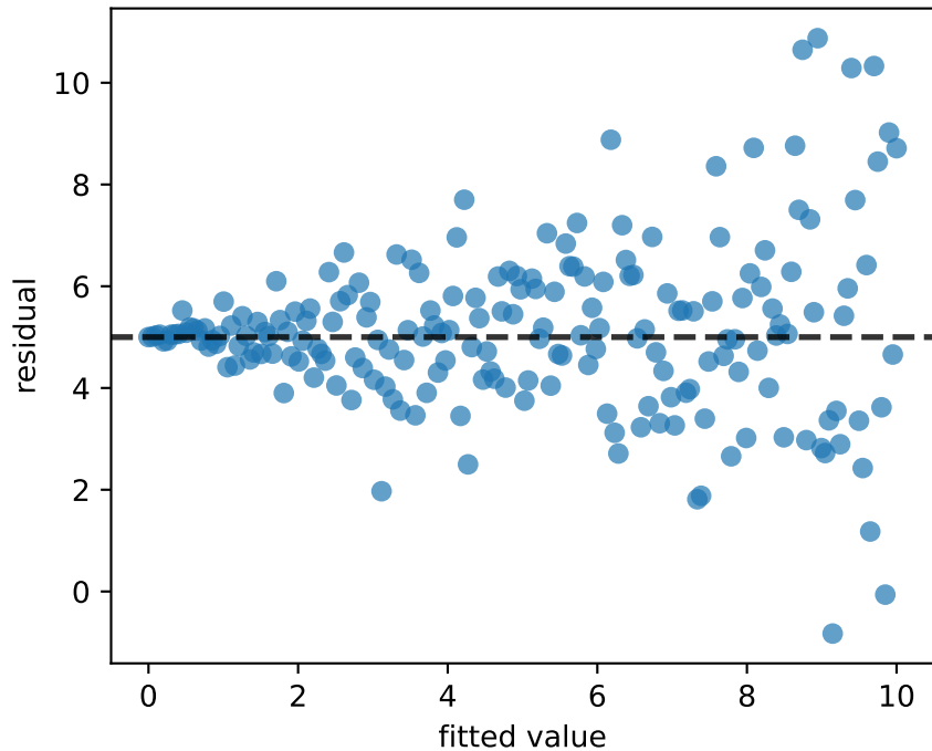
Heteroscedastic
