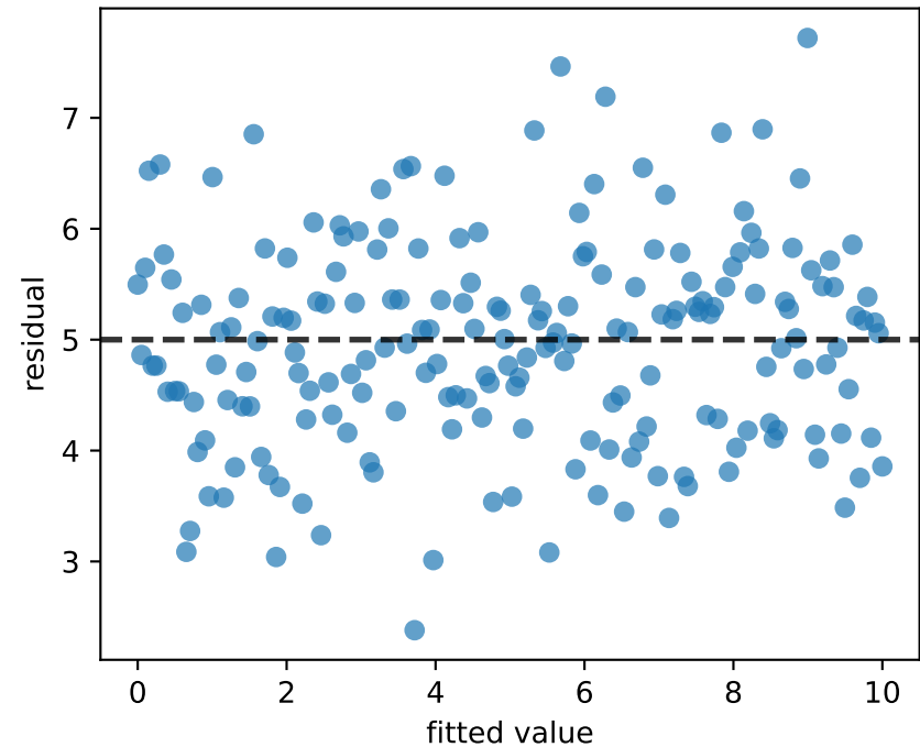
Homoscedastic
