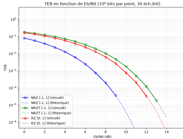
FIGURE 3.7 – TEB en fonction de E_b/N_0
