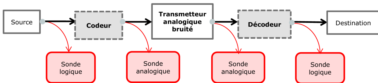
FIGURE 5.1 – Modélisation de la chaîne de transmission à l'étape 5a avec codage de canal.
