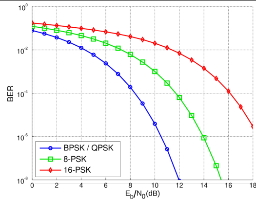
FIGURE 3.3 – Graphique du TEB par rapport au E_b/N_0 en fonction de la modulation. Source : Wikipédia.
