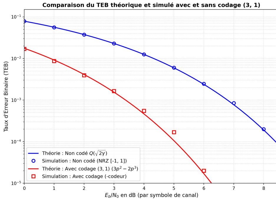
FIGURE 5.2 – Courbes de TEB en fonction de E_b/N_0 avec et sans codage de canal.
