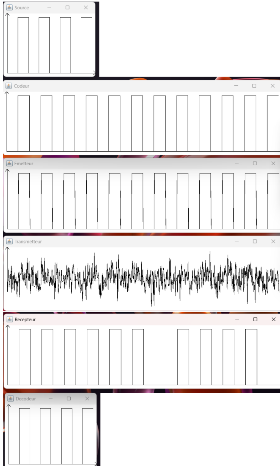
FIGURE 5.4 – Visualisation des sondes logiques et analogiques avec codage de canal. ./simulateur -mess 01010101 -s -form NRZ -snrpb 5 -codeur
