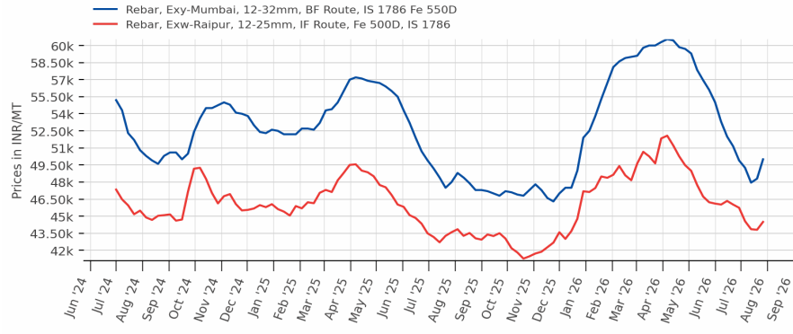
Rebar
