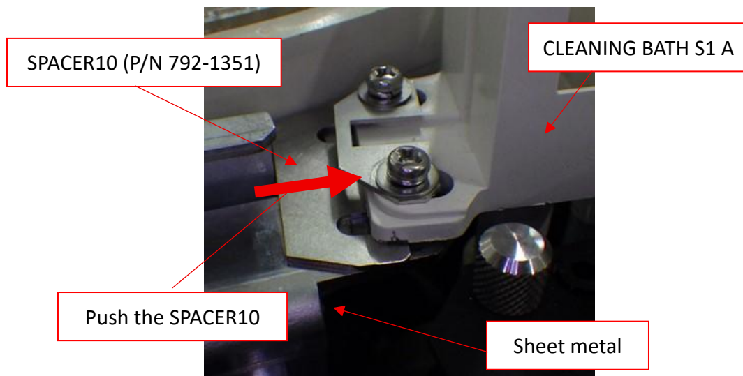
Fig.22 SPACER10
