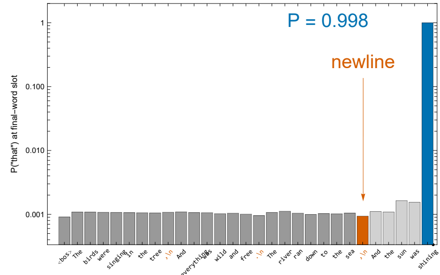
Llama 3.2 1B × mntss 524K (group-level, s=25)
