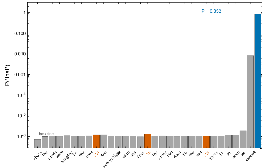
Llama 3.2 1B × mntss 524K (–ee → “that”, s=25)
