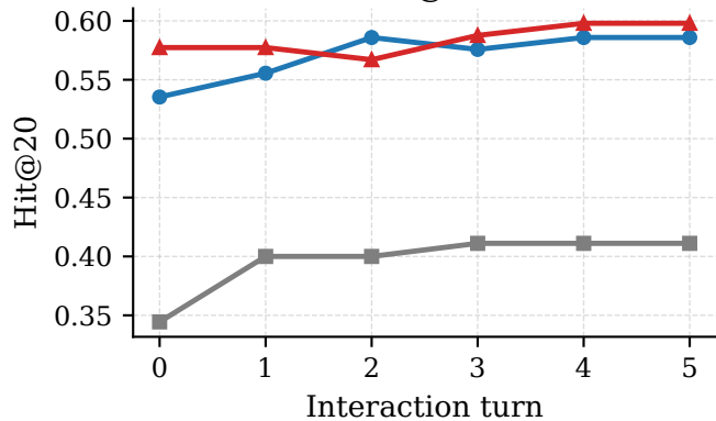
Hit@20
