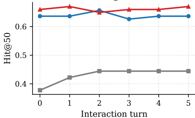
Hit@50
