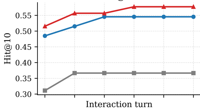
Hit@10
