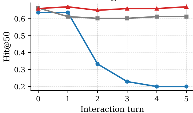
Hit@50
