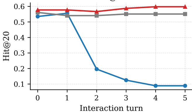
Hit@20
