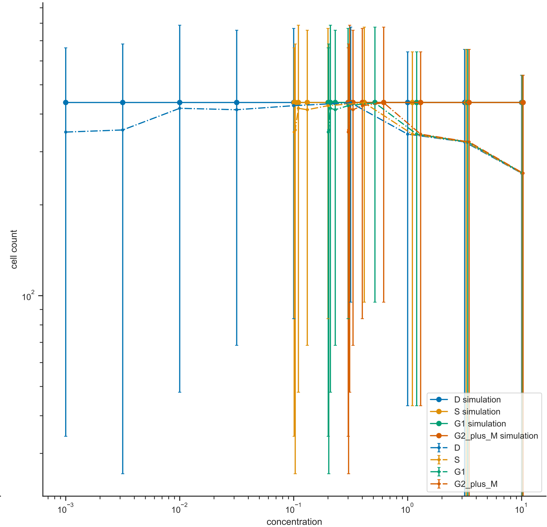
LEE011_Ribociclib
