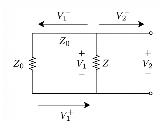
Fig. Solution Q3.07.1
