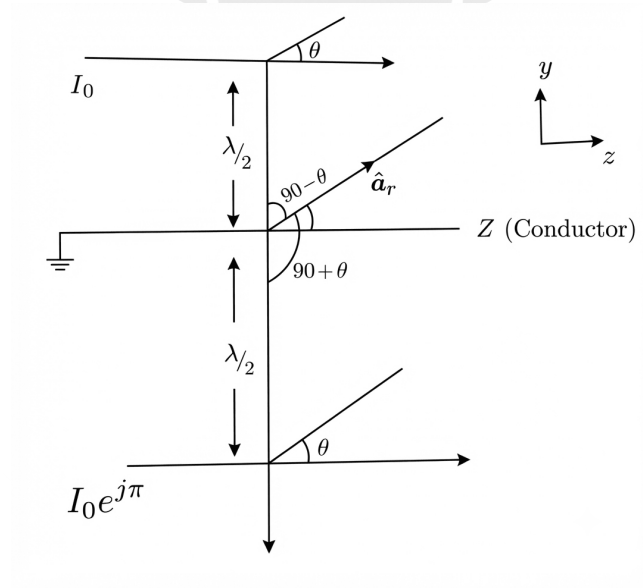
Fig. Solution Q5.07.1
