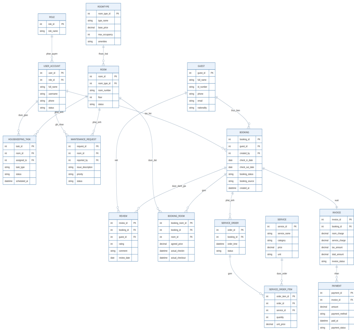
Hình 2. Sơ đồ ERD hệ thống HRMS
