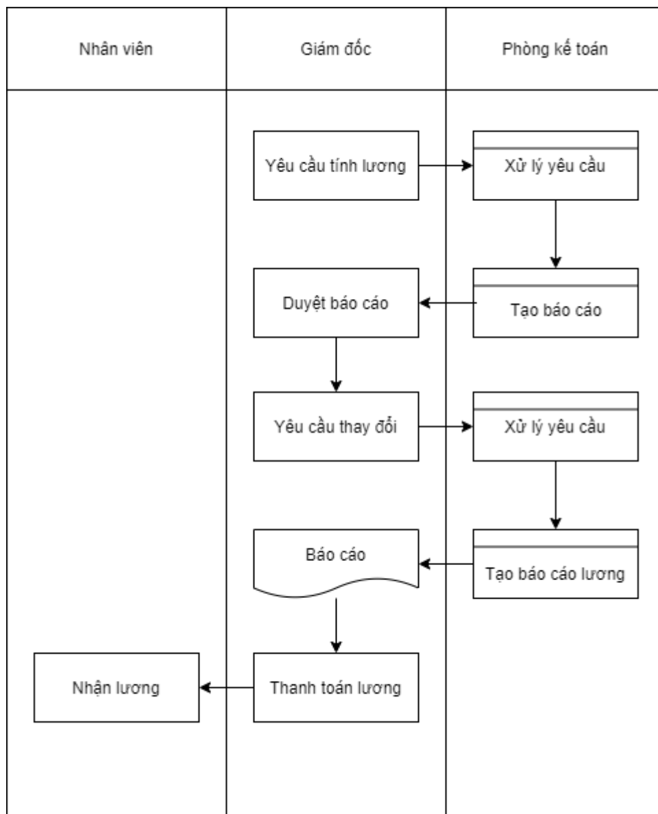
Hình 3.13: IFD Quản lý tính lương
