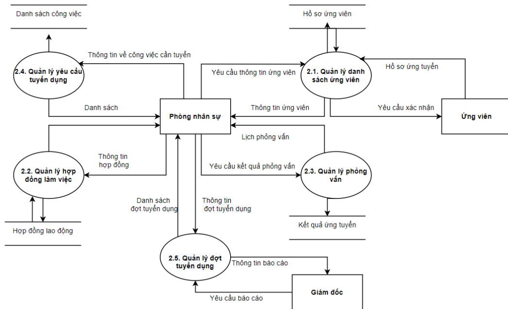
Hình 3.9: Sơ đồ luồng dữ liệu DFD mức 1 Quản lý tuyển dụng
