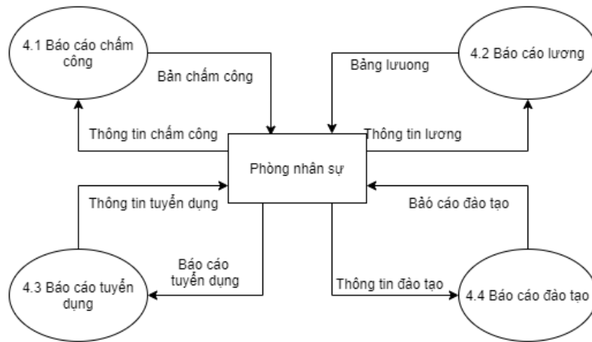
Hình 3.11: Sơ đồ luồng dữ liệu DFD mức 1 Báo cáo-thống kê
