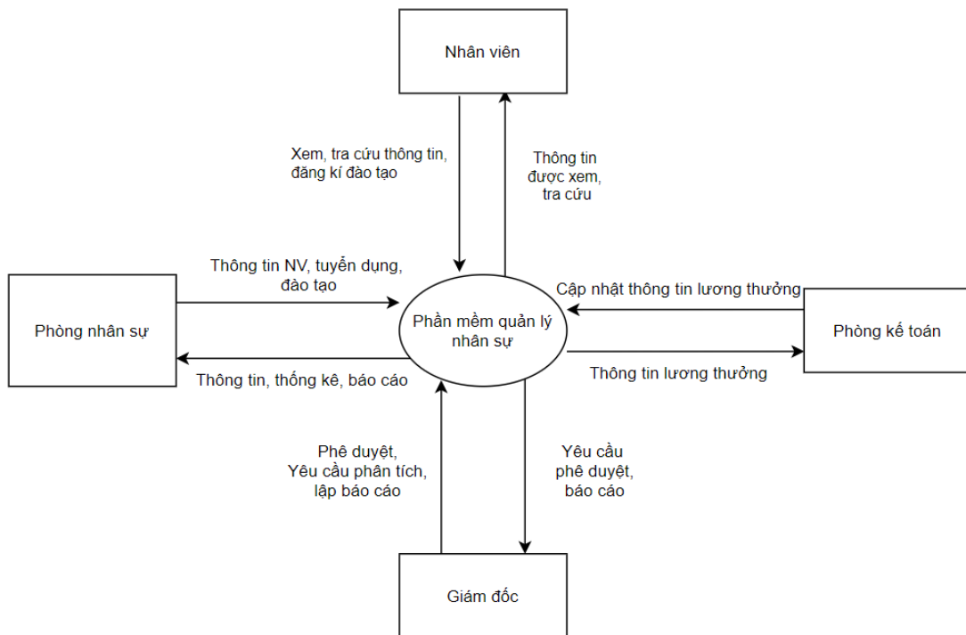
Hình 3.6: Sơ đồ ngữ cảnh CD
