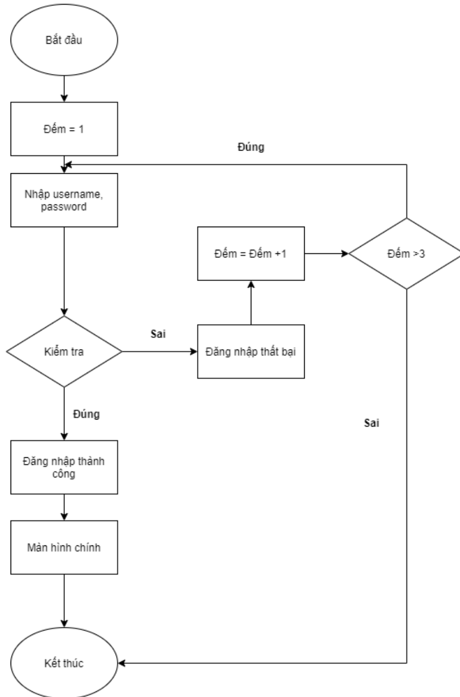
Hình 3.17: Giải thuật chức năng đăng nhập
