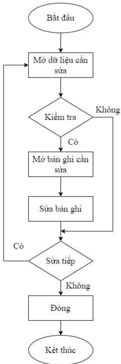
Hình 3.19: Giải thuật chức năng sửa dữ liệu
