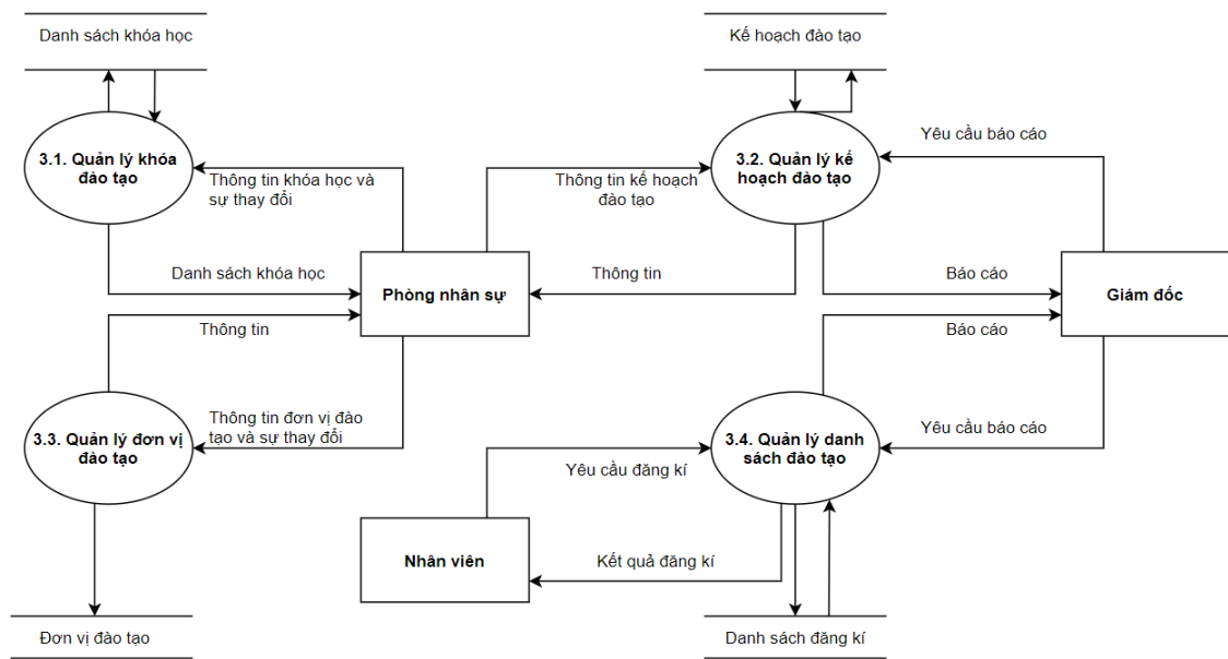
Hình 3.10: Sơ đồ luồng dữ liệu DFD mức 1 Quản lý đào tạo
