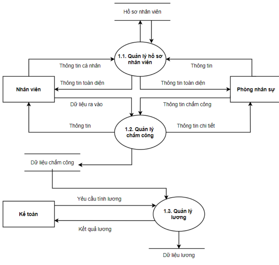
Hình 3.8: Sơ đồ luồng dữ liệu DFD mức 1 Quản lý nhân viên
