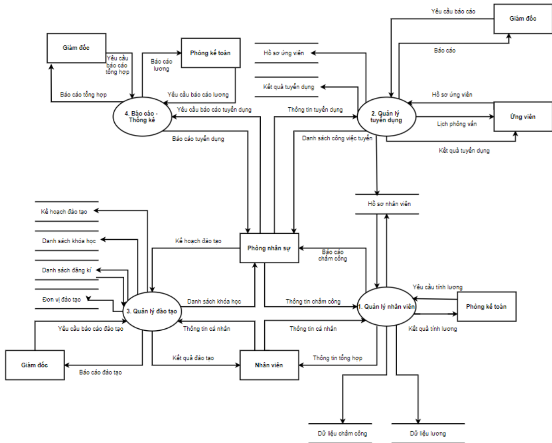
Hình 3.7: Sơ đồ luồng dữ liệu DFD mức 0
