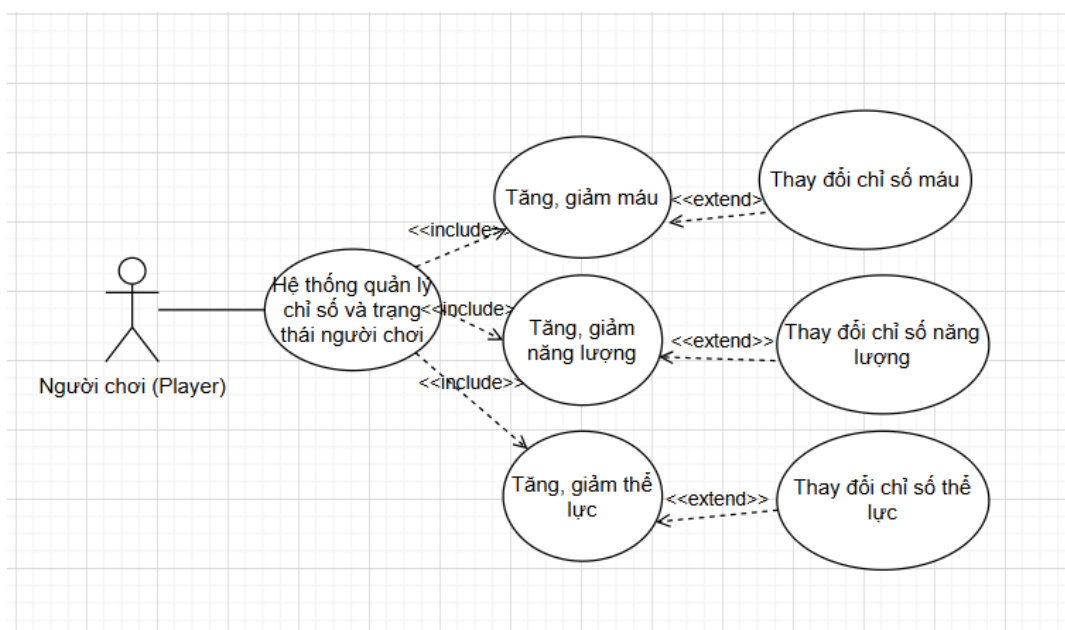
Biểu đồ 2.9. Biểu đồ use case hệ thống quản lý chỉ số và trạng thái người chơi
