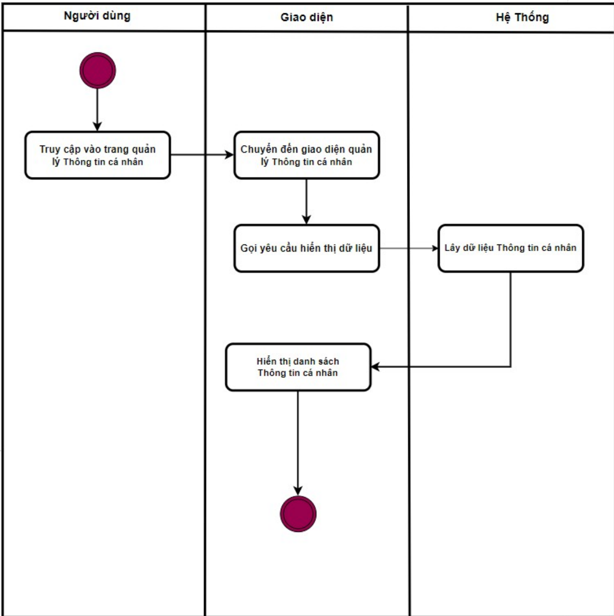
Hình 111: Biểu đồ hoạt động “Chức năng danh sách thông tin cá nhân”
