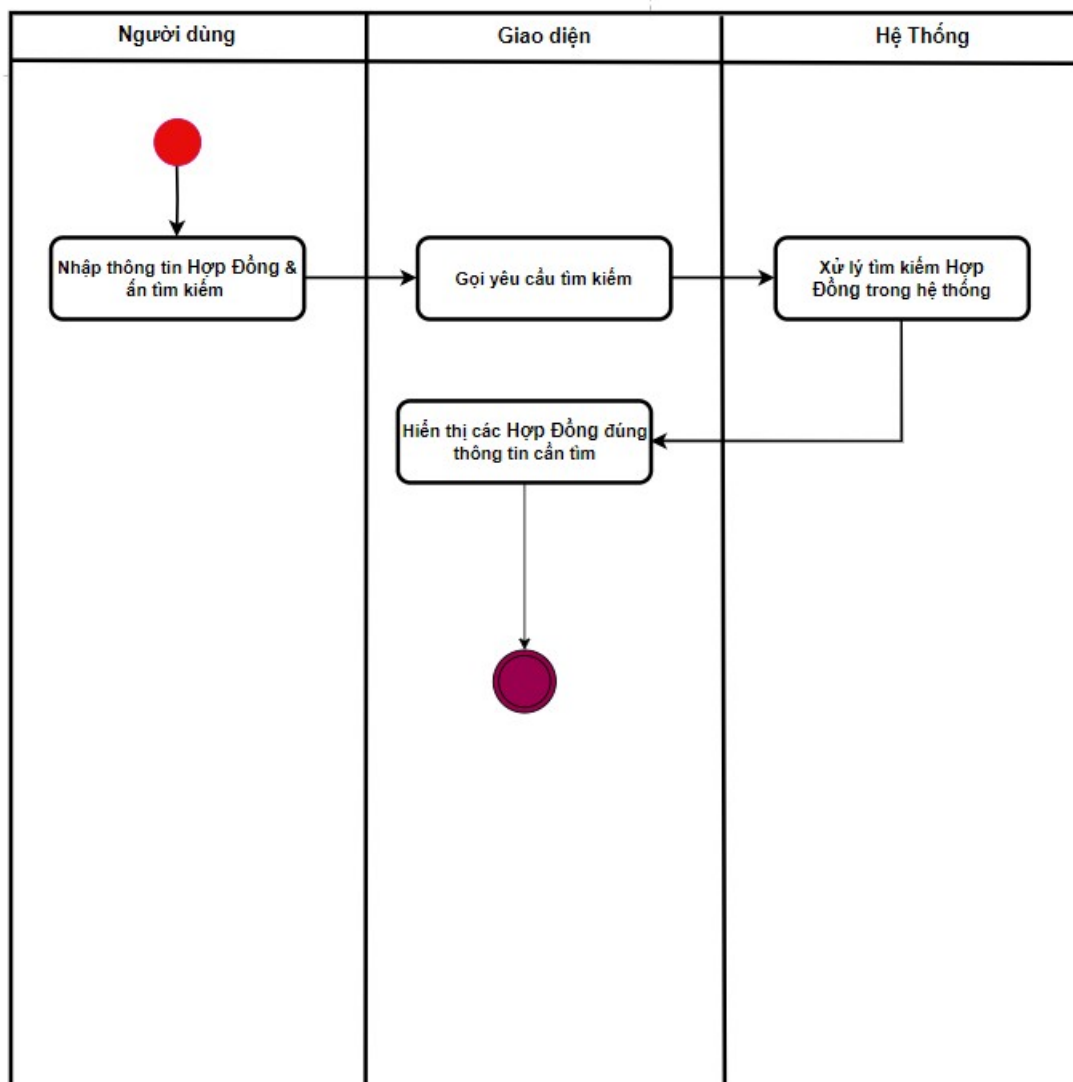
Hình 88: Biểu đồ hoạt động “Chức năng tìm kiếm hợp đồng”
