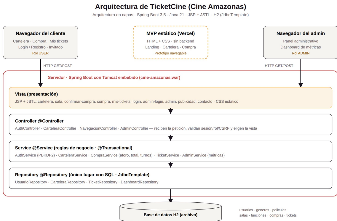
Figura 12. Arquitectura en capas de TicketCine.
