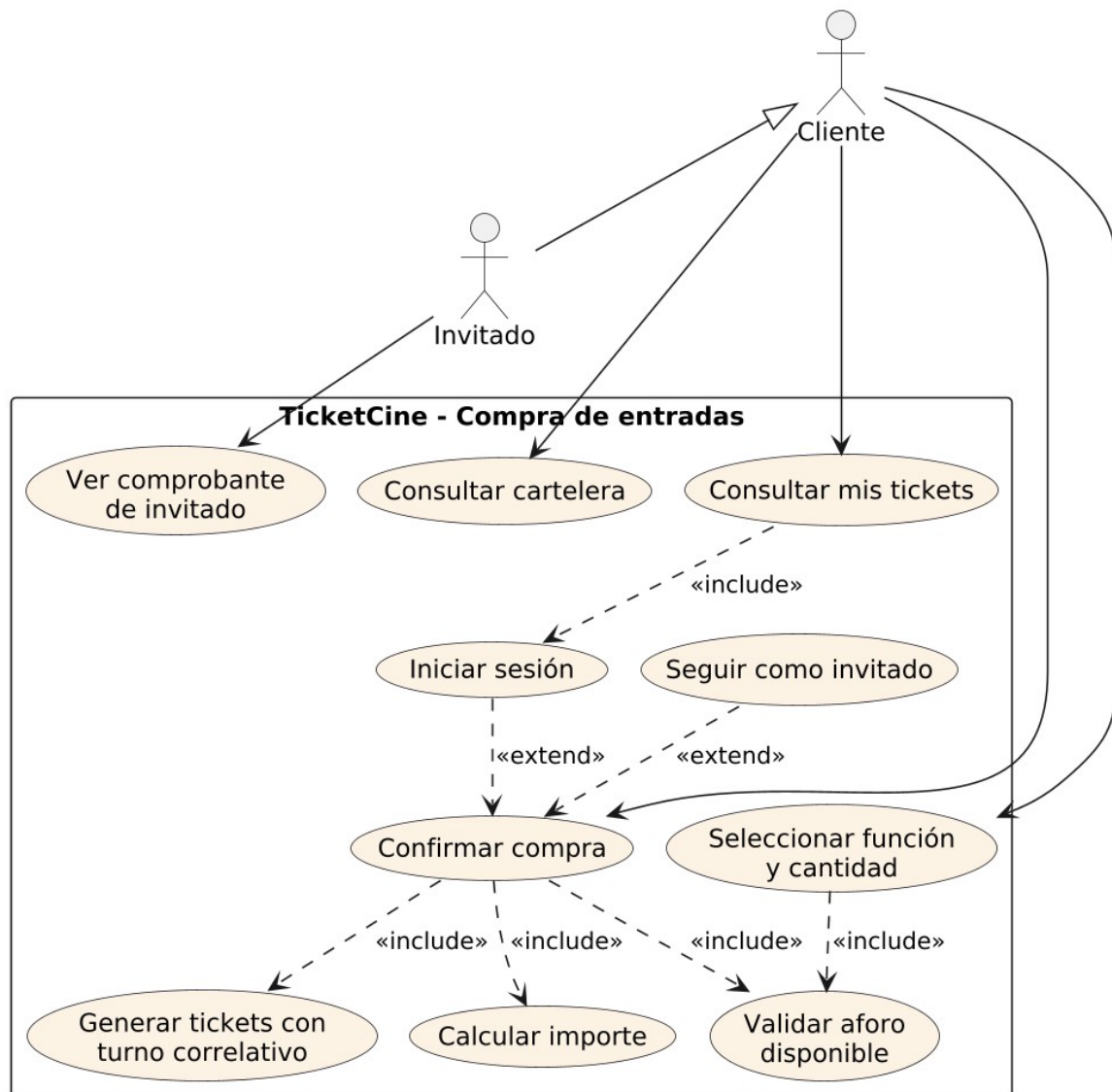
Figura 10. Casos de uso del proceso core (fuente: docs/diagramas/cu-core.puml).
