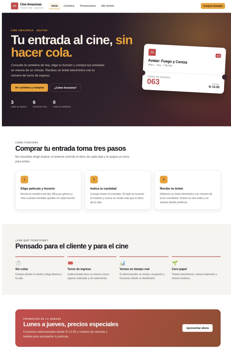
Figura 19. Landing page de TicketCine construida solo con HTML5 y CSS3 (archivo mvp/index.html).
