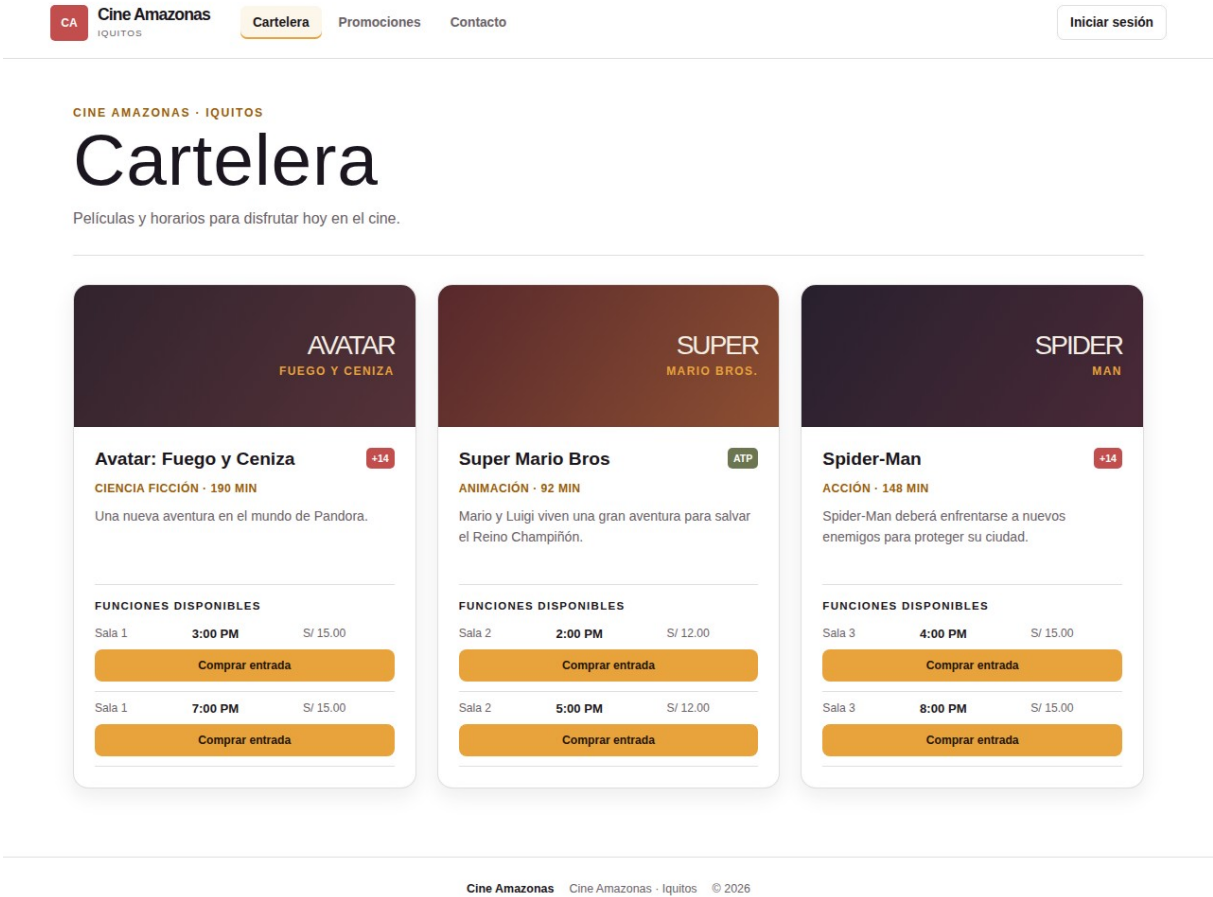
Figura 1. Interfaz Cartelera (aplicación Spring Boot).
