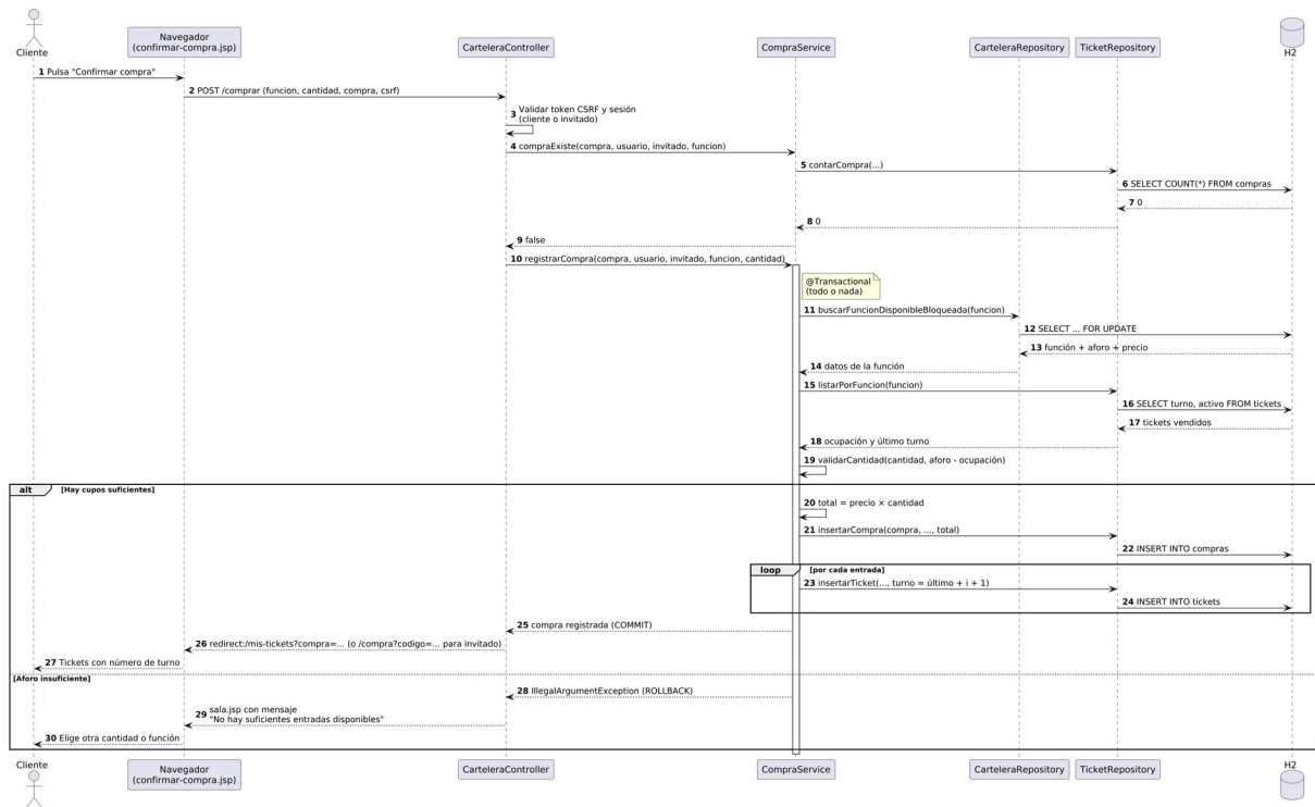
Figura 8. Diagrama de secuencia del proceso core (fuente: docs/diagramas/sec-core.puml).
