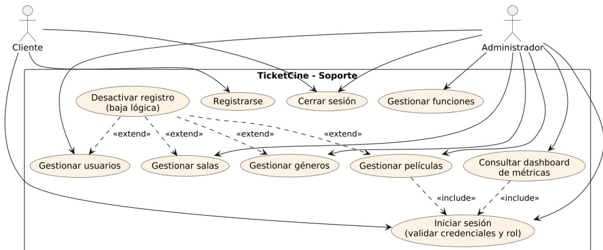
Figura 11. Casos de uso de los procesos de soporte (fuente: docs/diagramas/cu-soporte.puml).
