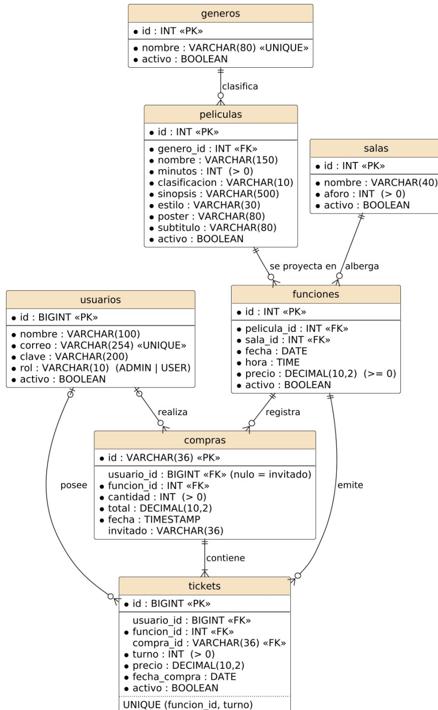
Figura 7. Diagrama entidad-relación de TicketCine (fuente: docs/diagramas/er.puml).
