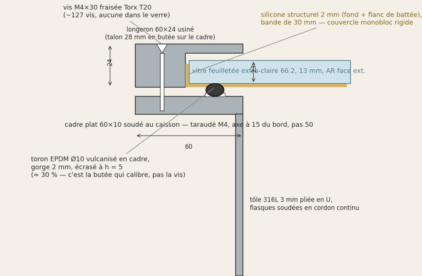
02 — Détail du serrage périphérique : longeron à battée (cotes en mm)
