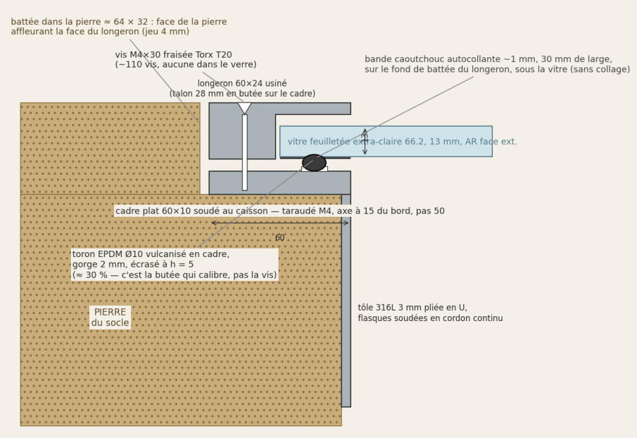
02 — Détail du serrage périphérique dans la battée de pierre (cotes en mm)
