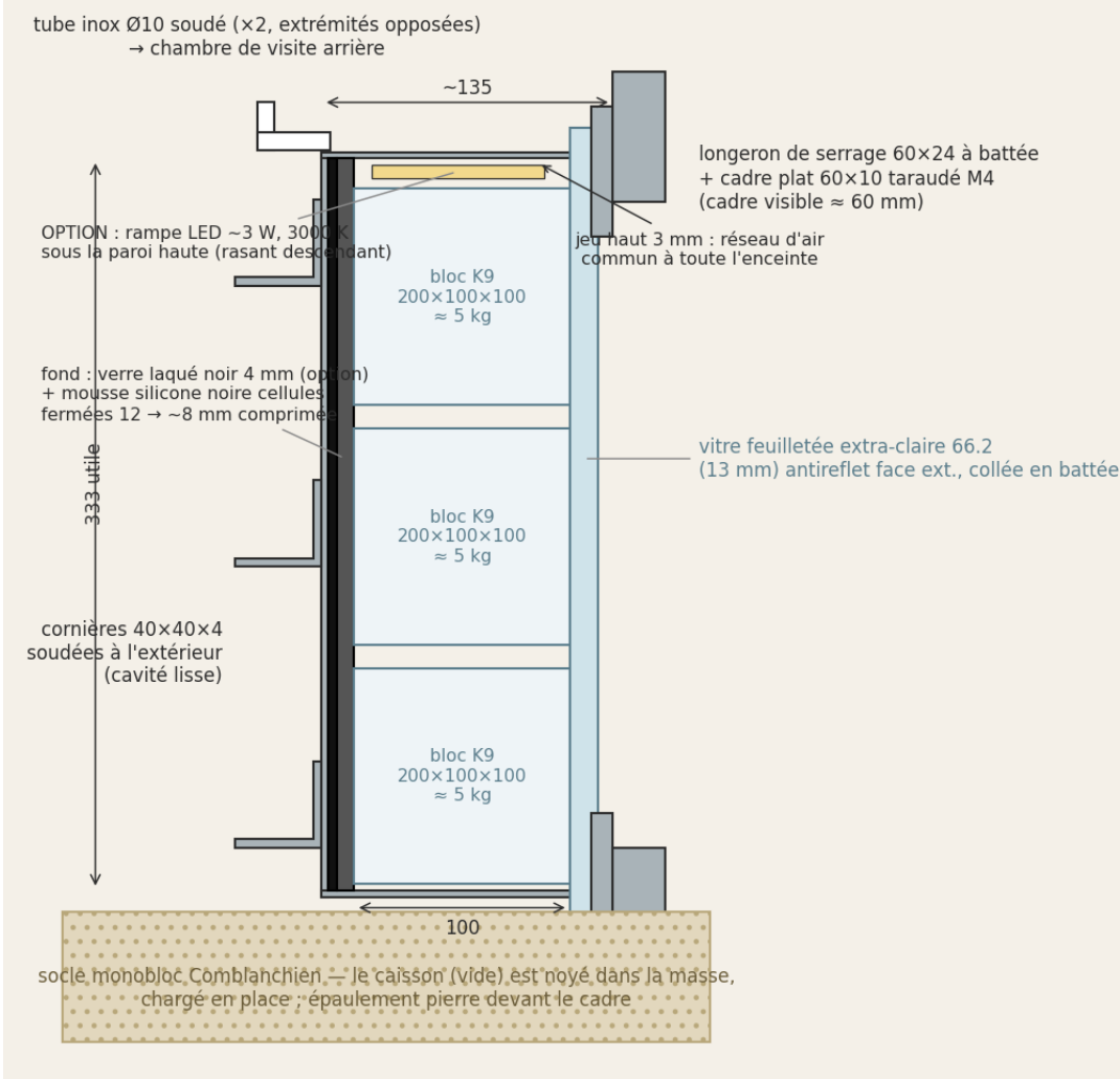
01 — Coupe verticale de principe (cotes en mm, échelle indicative)
