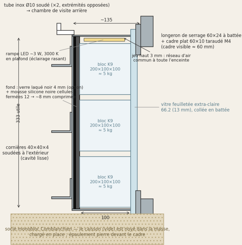
02 — Détail du serrage périphérique : longeron à battée (cotes en mm)
