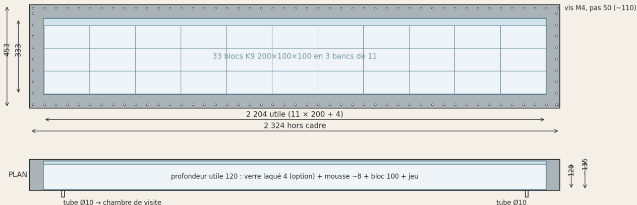
03 — Vue de face et plan cotés, 3 × 11 blocs (mm)
