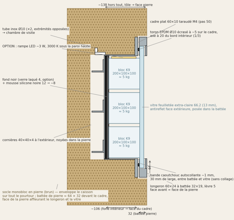
02 — Détail du serrage périphérique dans la battée de pierre (cotes en mm)
