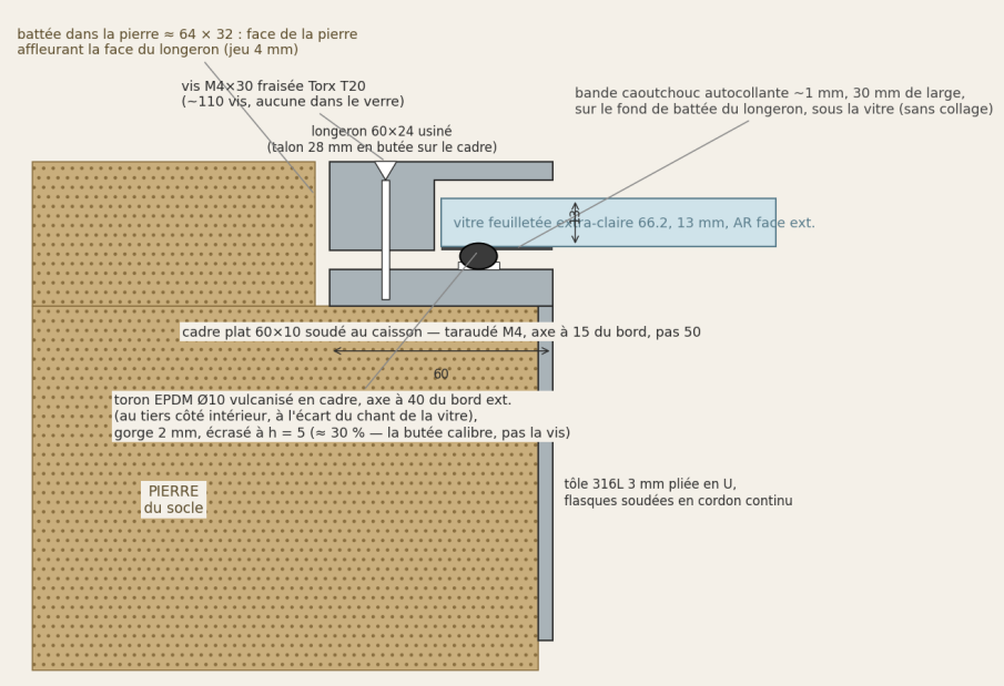
02 — Détail du serrage périphérique dans la battée de pierre (cotes en mm)
