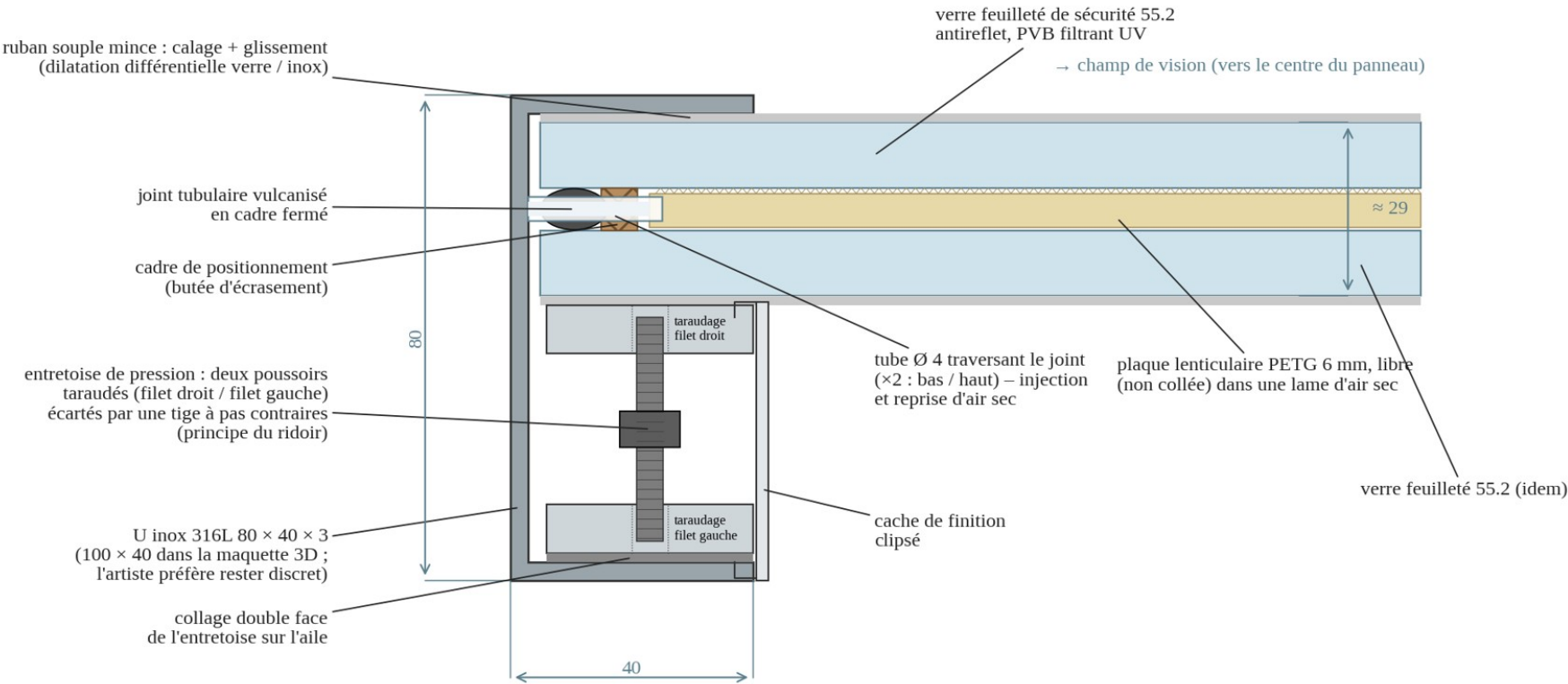
Coupe horizontale dans un montant – principe du serrage périphérique (échelle ≈ 1:1, cotes en mm)
