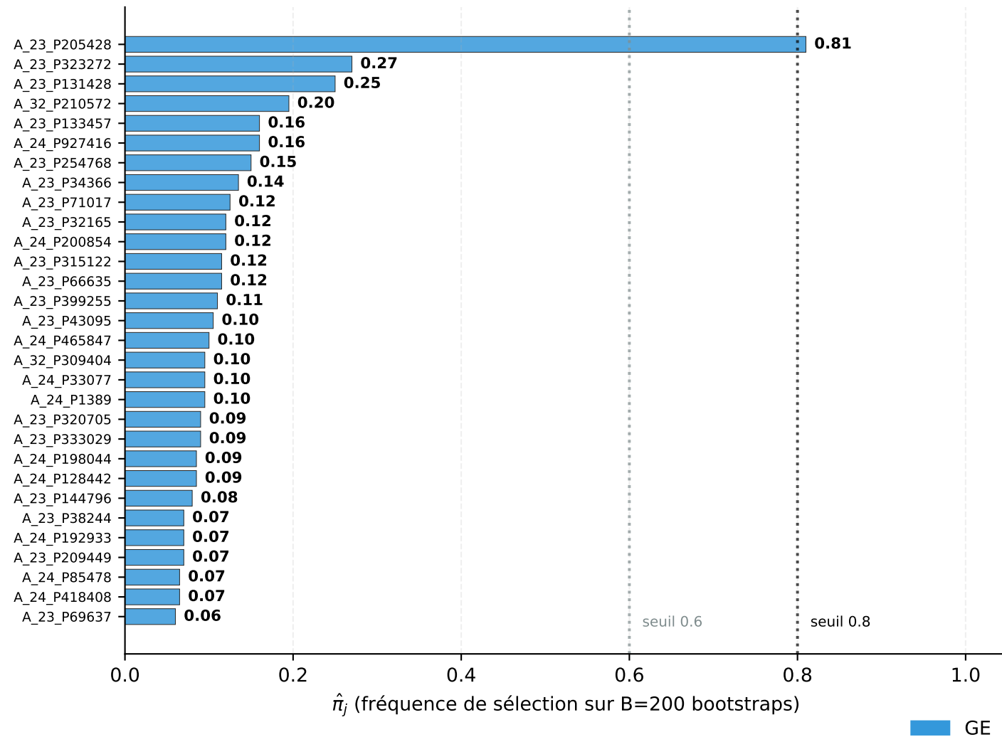
OvR binomial Lasso
