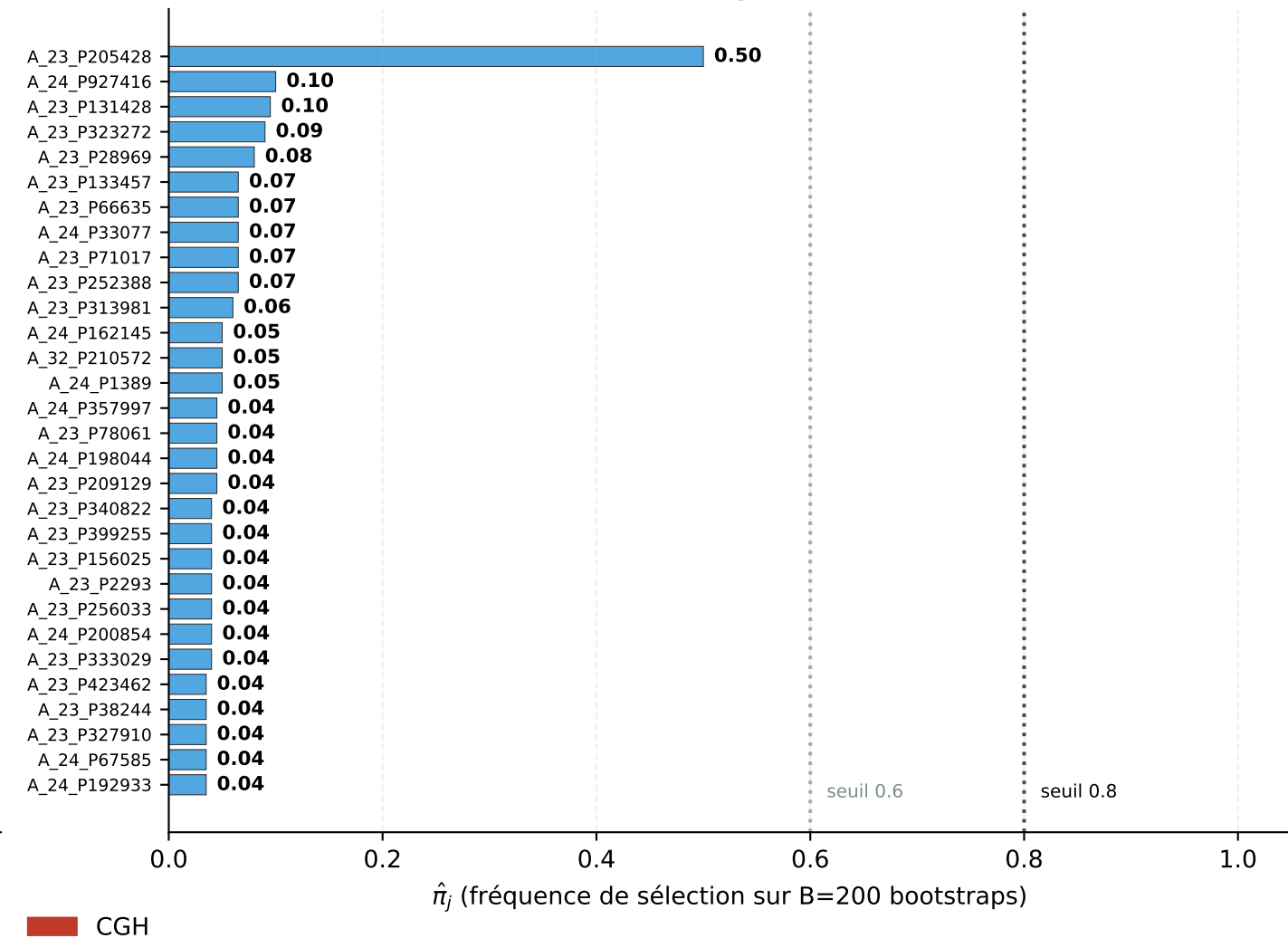
Multinomial ungrouped Lasso
