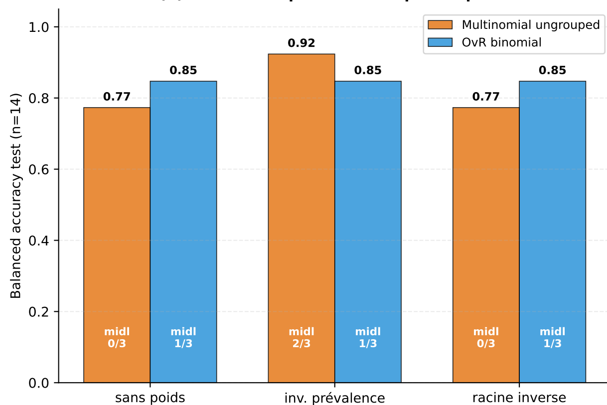
(B) Test — récupération midl par les poids
