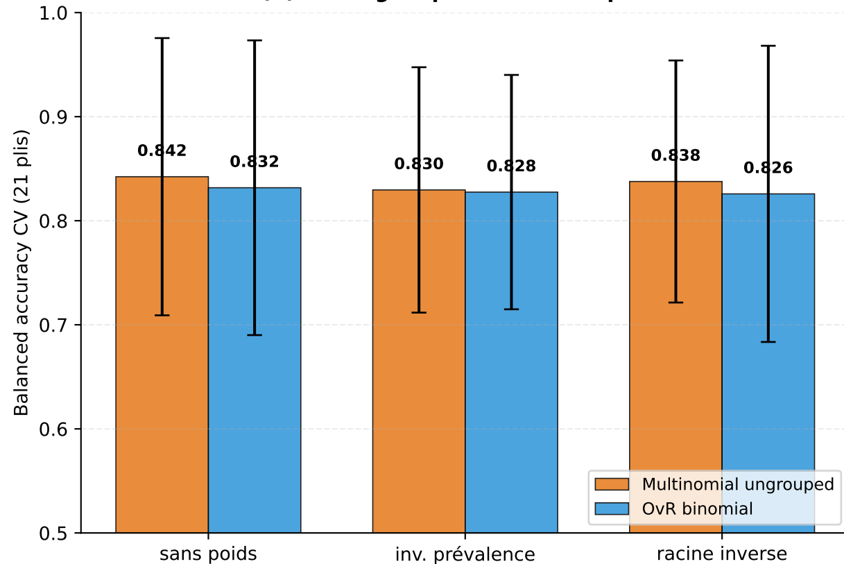
(A) CV — gain par schéma de poids
