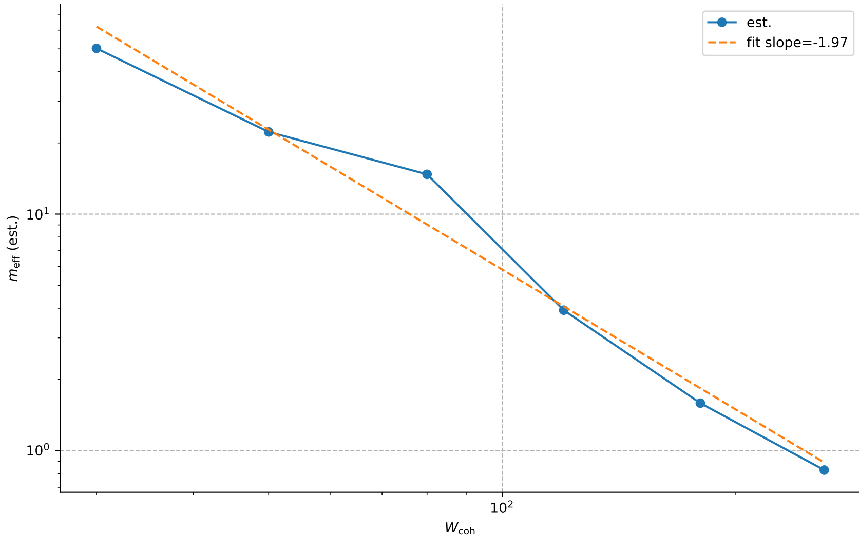
Fig. 3 m_{\text{eff}} vs W_{\text{coh}}
