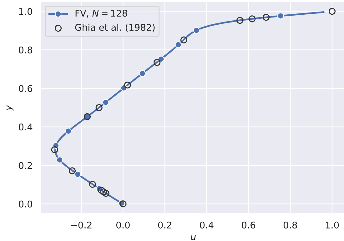
u -velocity (vertical centerline)
