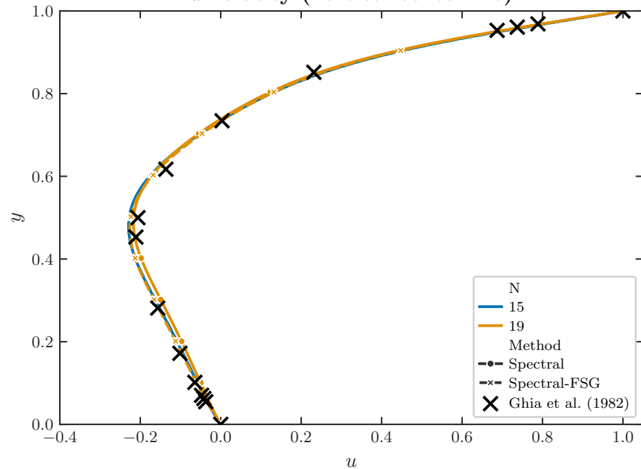
u -velocity (vertical centerline)
