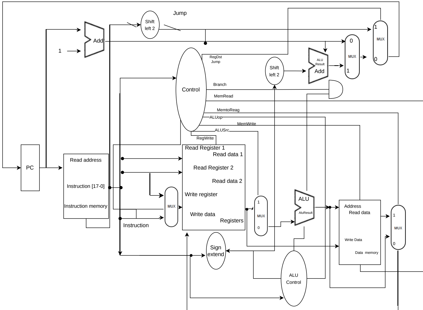
Diagrama de bloco - Processador MIPS de 8 bits (ciclo único)
