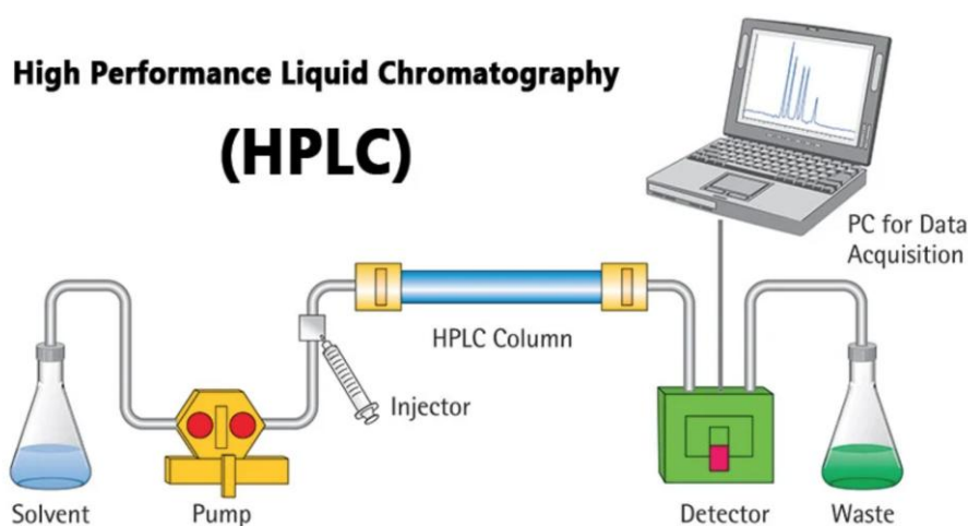
Figure 70.principe de fonctionnement de l'HPLC 412
