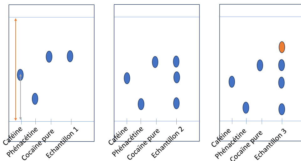
Figure 68. Exemple de CCM d'échantillons de cocaïne
