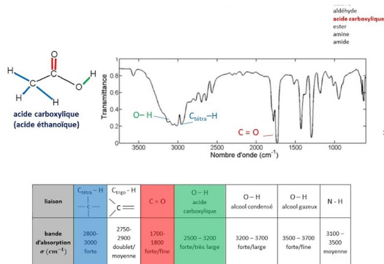
Figure 69. Exemple de spectre infrarouge 411
