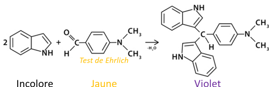
Figure 64. Exemple du test de Ehrlich permettant de détecter du LSD.
