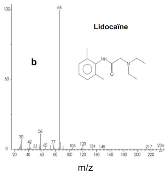
Figure 73. Exemple de spectre de masse pour la molécule de Lidocaïne 413
