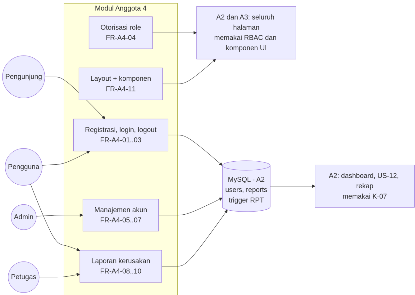
Diagram 1 — 2.1 Perspektif produk
