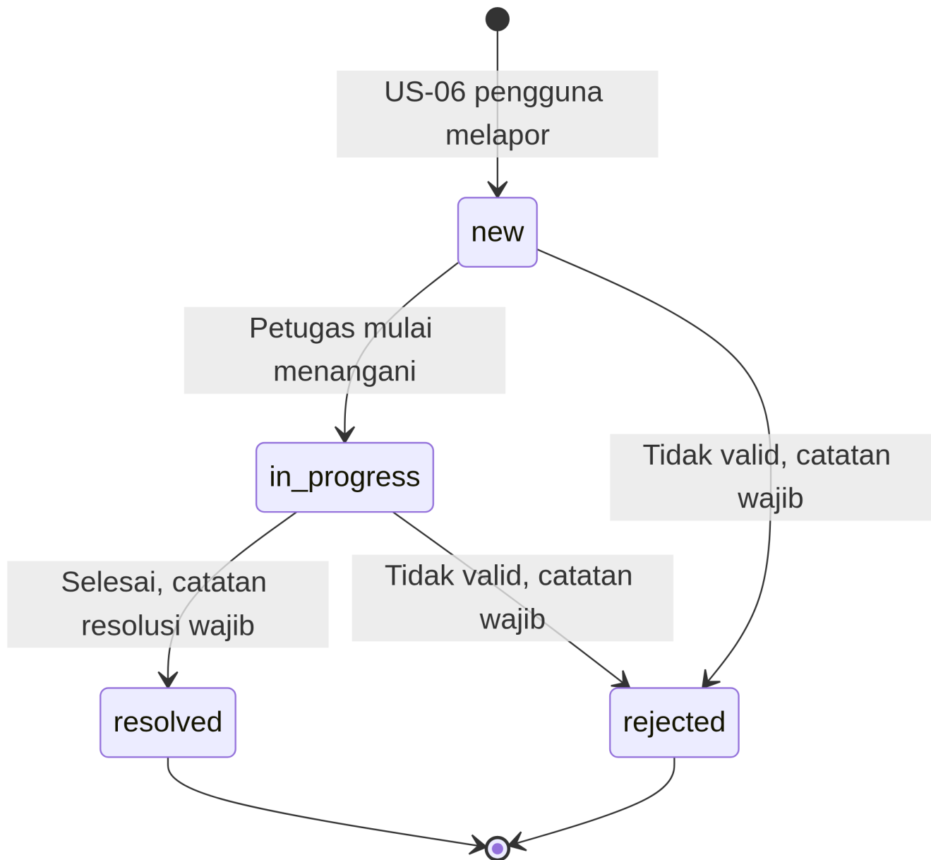
Diagram 4 — 8.2 Siklus hidup laporan (FR-A4-08..10)
